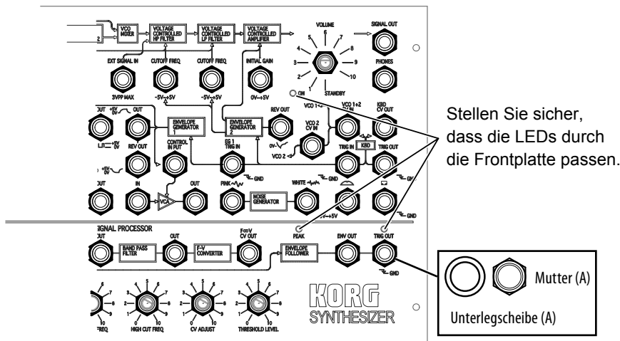
Buchsenfeldplatine
