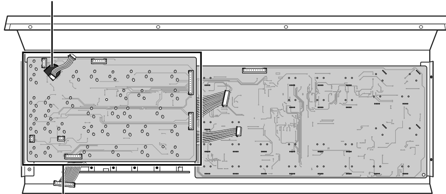
Buchsenfeldplatine
