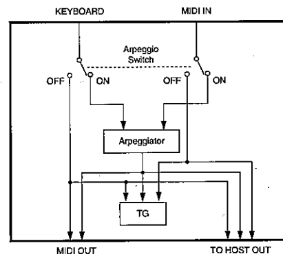
図はローカルON、グローバル・パラメータのPC I/TO PORT=Emulateの場合です。
