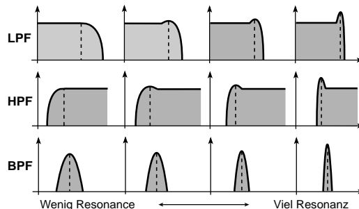
Funktionsprinzip von Resonance
