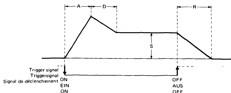
"ADSR"-Hüllkurvensignal
