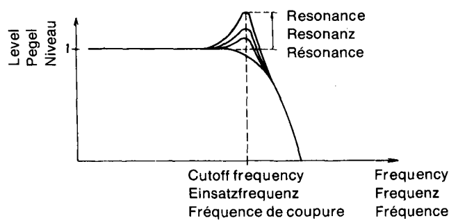
VCF-Frequenzempfindlichkeit
