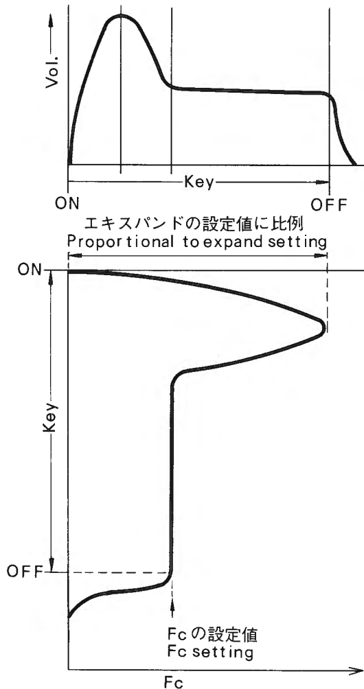
fig. 45 The EXPAND of woodwind instrument. (木管楽器のエキスパンド)
