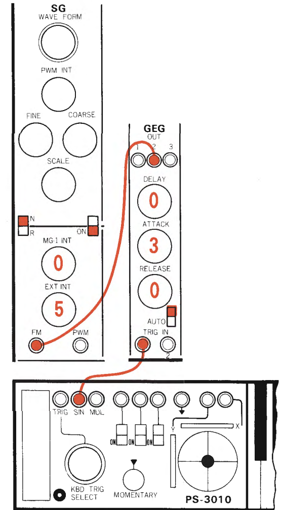
fig.27 Pitch bend (ベンダー・アップ)
