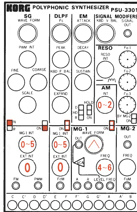
fig. 47 Vibrato (ビブラート効果)
