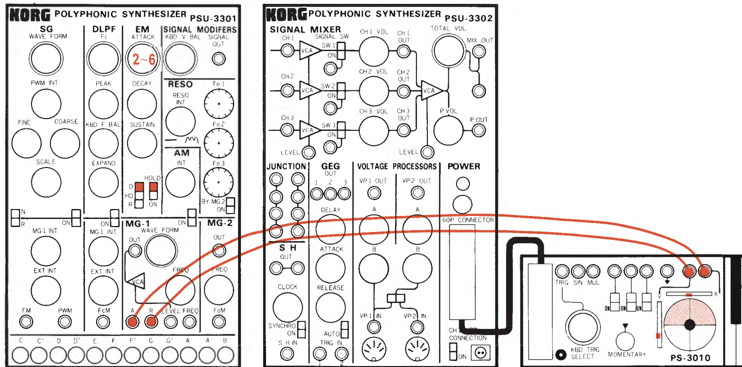
fig. 53 Manual control of envelope. (手もとで、音量変化をコントロールする場合)
