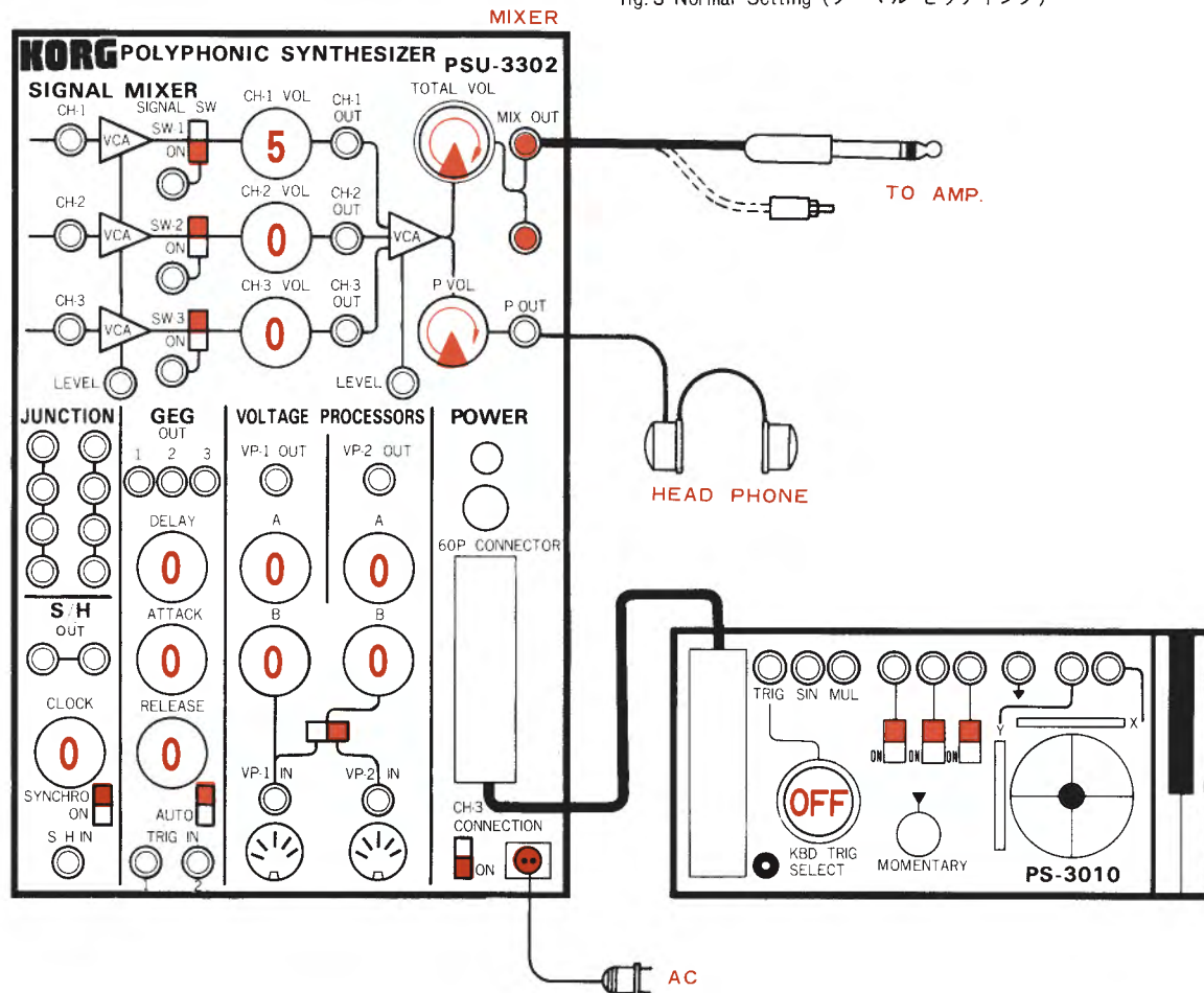
fig.3 Normal Setting (ノーマル・セッティング)
