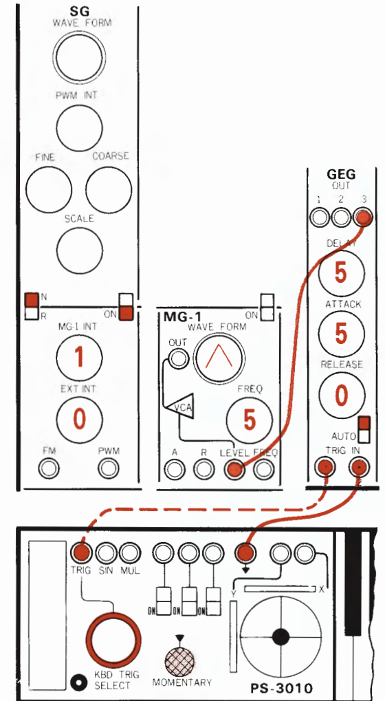
fig.30 Momentary vibrato (モーメンタリー・ビブラート)
