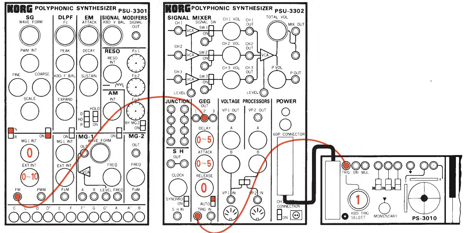
fig.48 Bend (ベンド効果)
