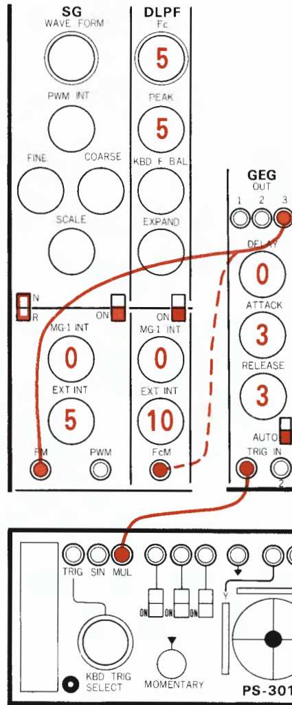
fig.29 Multiple trigger bend (マルチ・ベンド)
