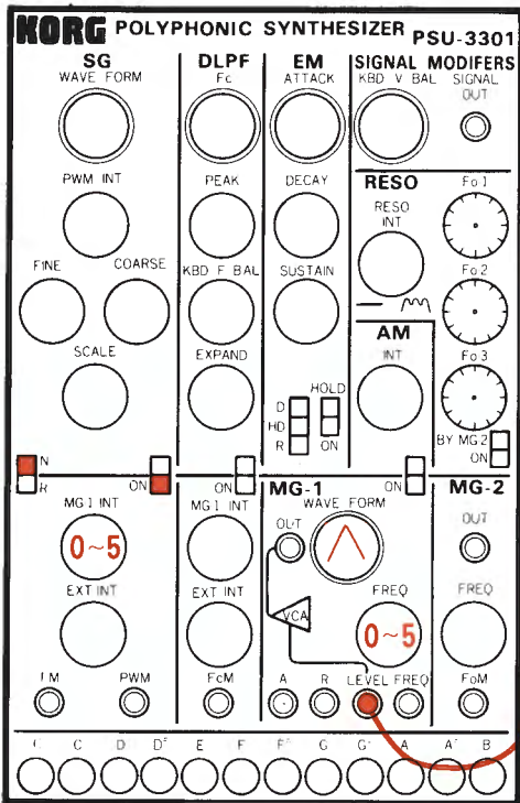
fig. 49 Delayed vibrato (テイレイ・ビブラトを得る場合)
