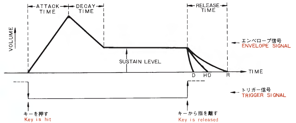
fig. 8 Envelope Signal (エンベロープ信号)
