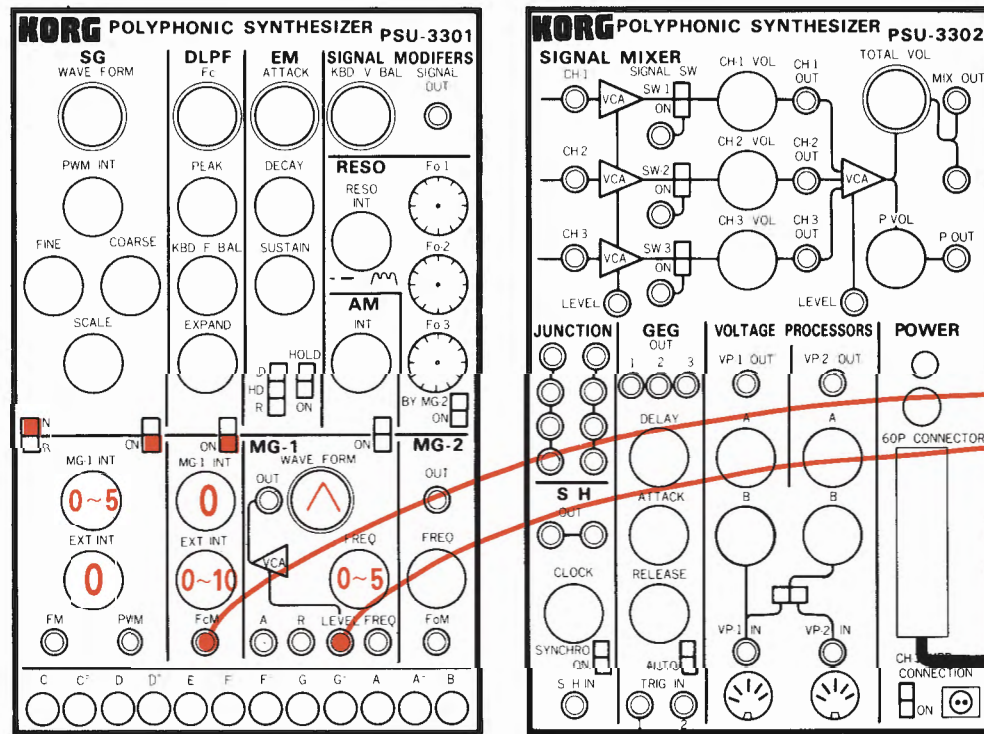
fig.51 Manual control of both tone color and vibrato depth. (手もとで、ビブラートの深さと音色をコントロールする場合)
