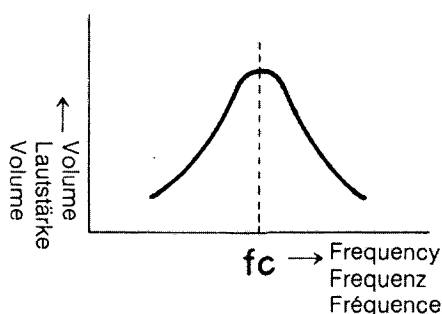
Band-pass filter characteristics. Eigenschaften des Bandpaßfilters. Caractéristiques du filtre passe-bande.
